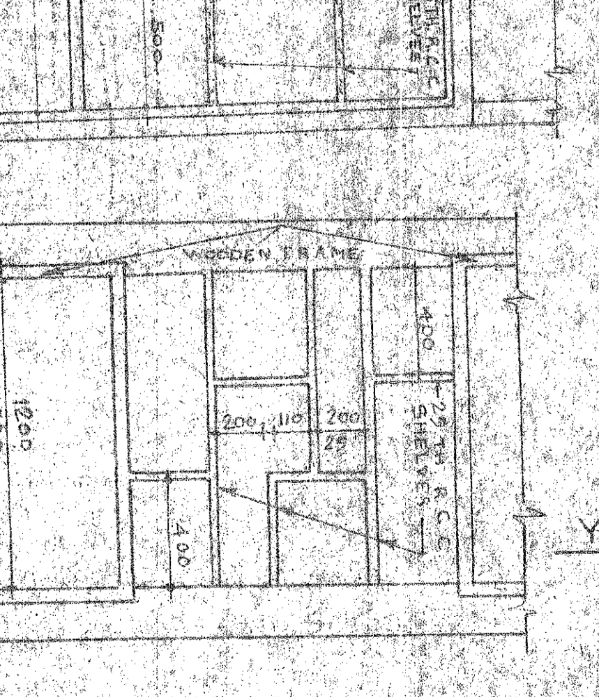
SECTION D-D
